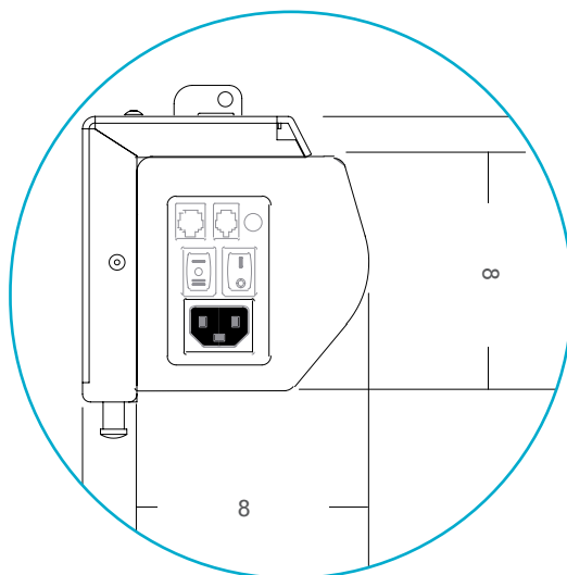
Côté du carter avec patte de fixation Side of the case with bracket
