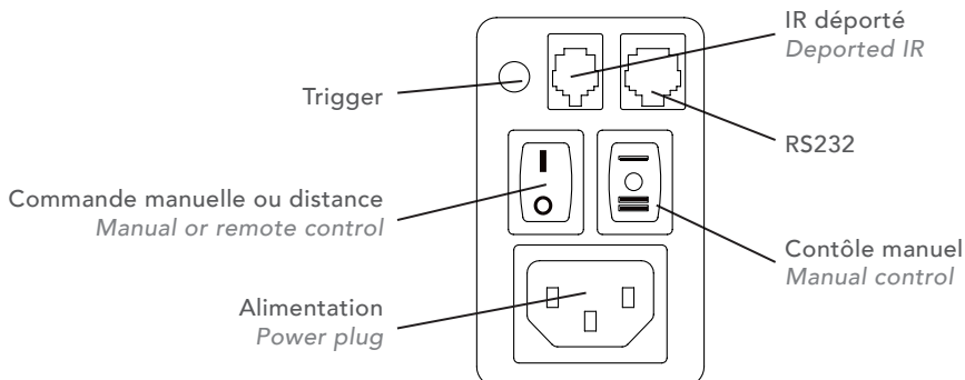
Panneau de contrôle Control panel
