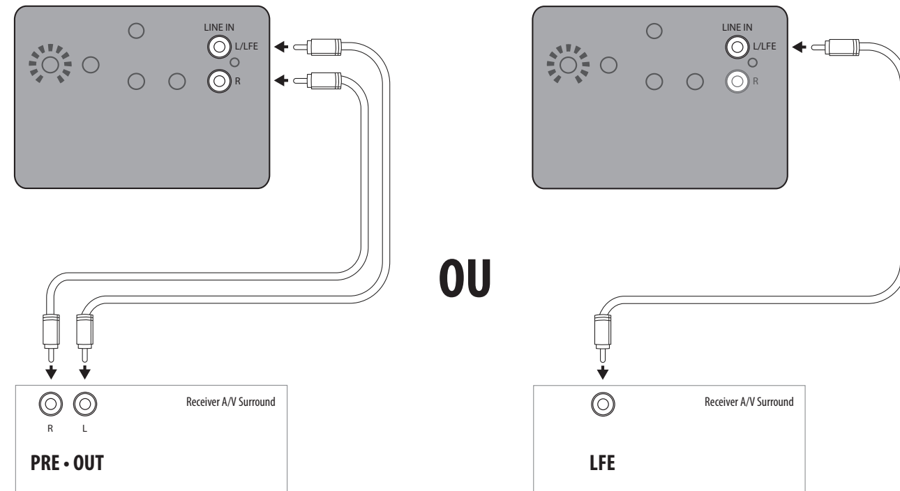
Figura 2 Conexão Do Subwoofer J 110, J 112
