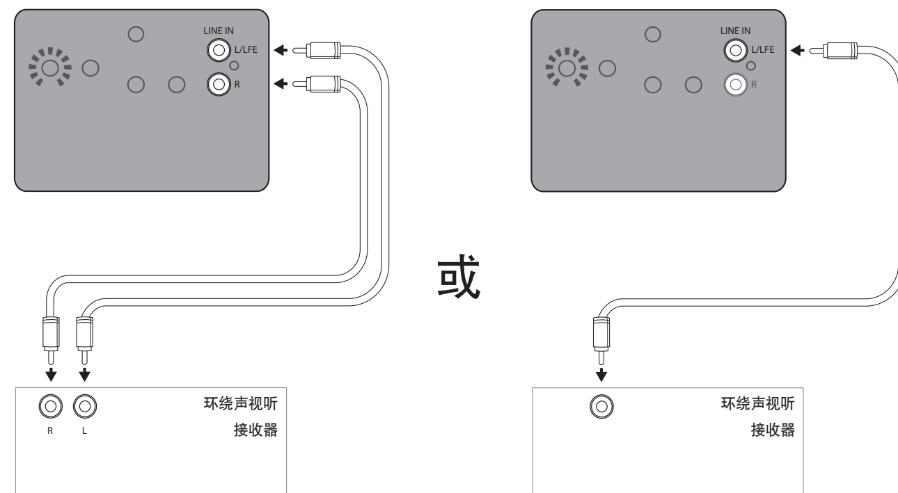
图2 J 110、J 112低音炮连接图
