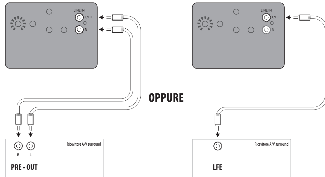
Figura 2 Connessioni Di Un Subwoofer J 110, J 112
