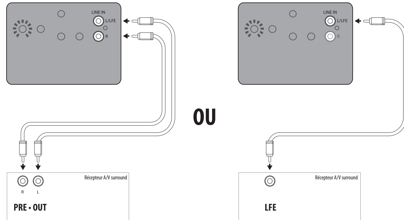
Figure 2 Branchement D'un Caisson De Graves J 110, J 112
