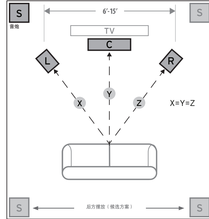
图1 聆听区的音箱摆放方式
