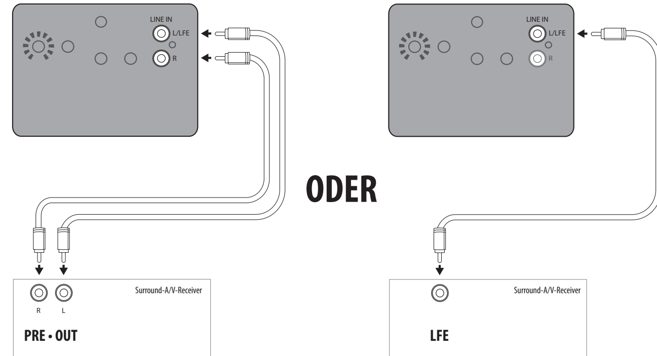
Abbildung 2 Anschluss Für Den Subwoofer J 110, J 112
