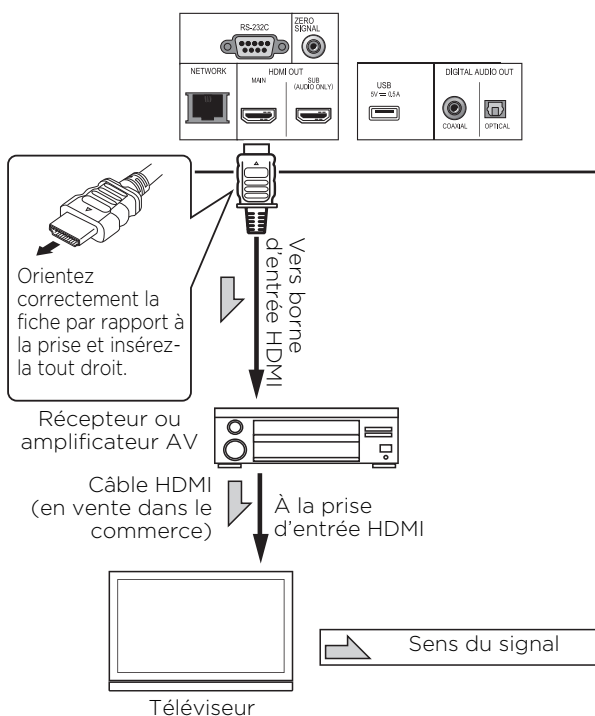
Face arrière du UDP-LX500
