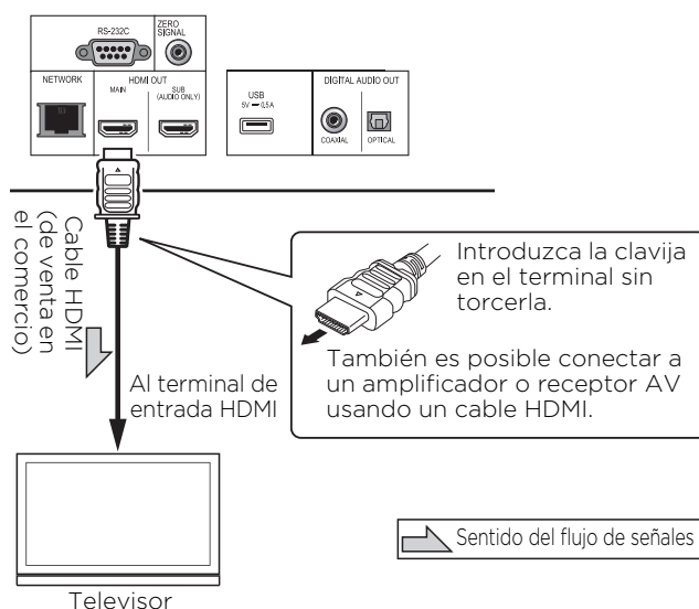
Panel posterior de UDP-LX500
