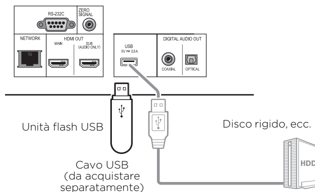
Pannello posteriore del UDP-LX500
