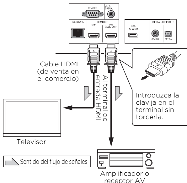
Panel posterior de UDP-LX500
