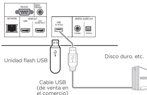
Panel posterior de UDP-LX500
