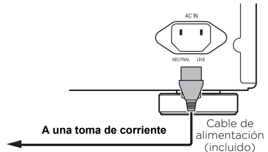
Panel posterior de UDP-LX500
