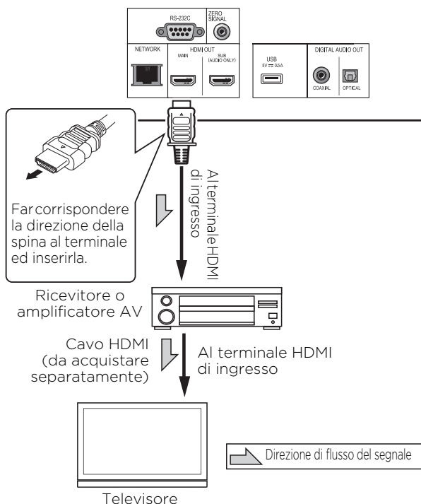
Pannello posteriore del UDP-LX500
