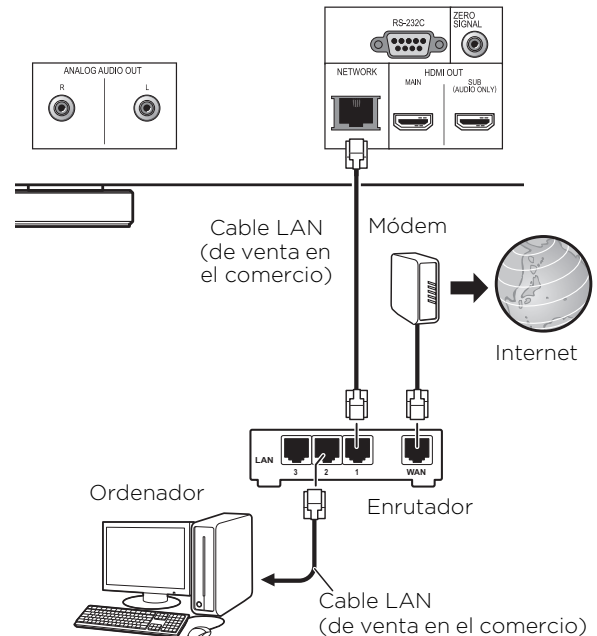
Panel posterior de UDP-LX500
