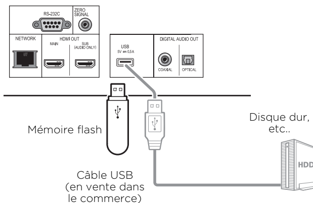
Face arrière du UDP-LX500
