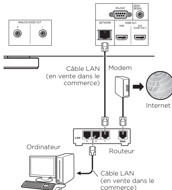
Face arrière du UDP-LX500
