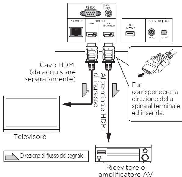
Pannello posteriore del UDP-LX500
