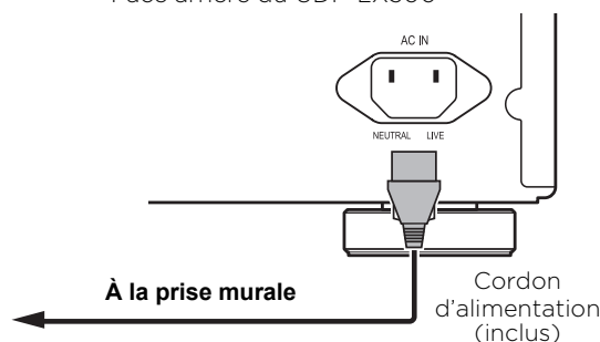
Face arrière du UDP-LX500
