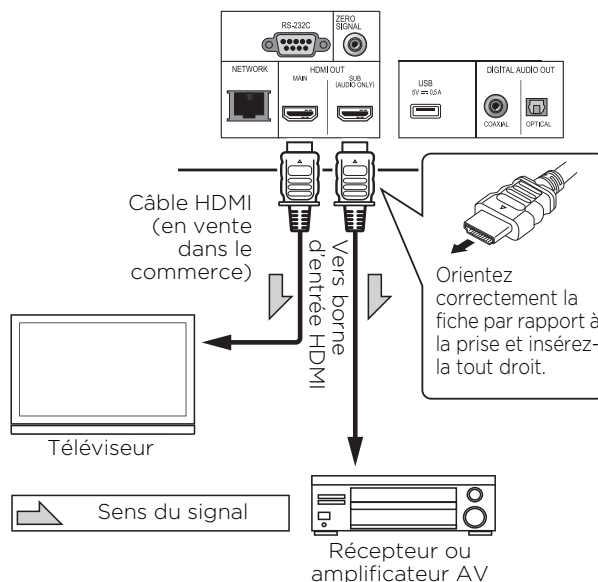
Face arrière du UDP-LX500
