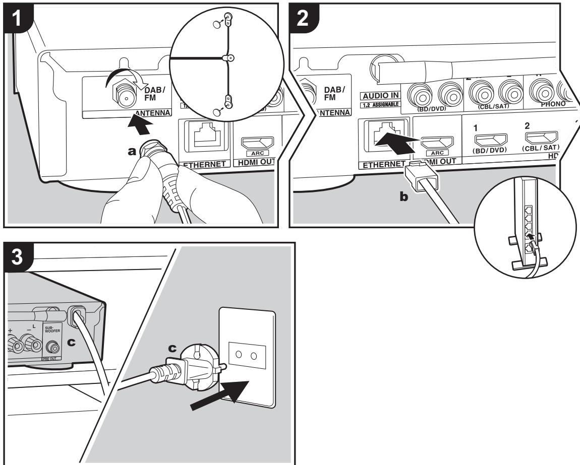
a DAB/FM-antenne, b Ethernet-kabel, c Netsnoer
