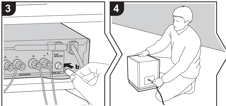
a Câble d'enceinte, b Câble du caisson de basse
